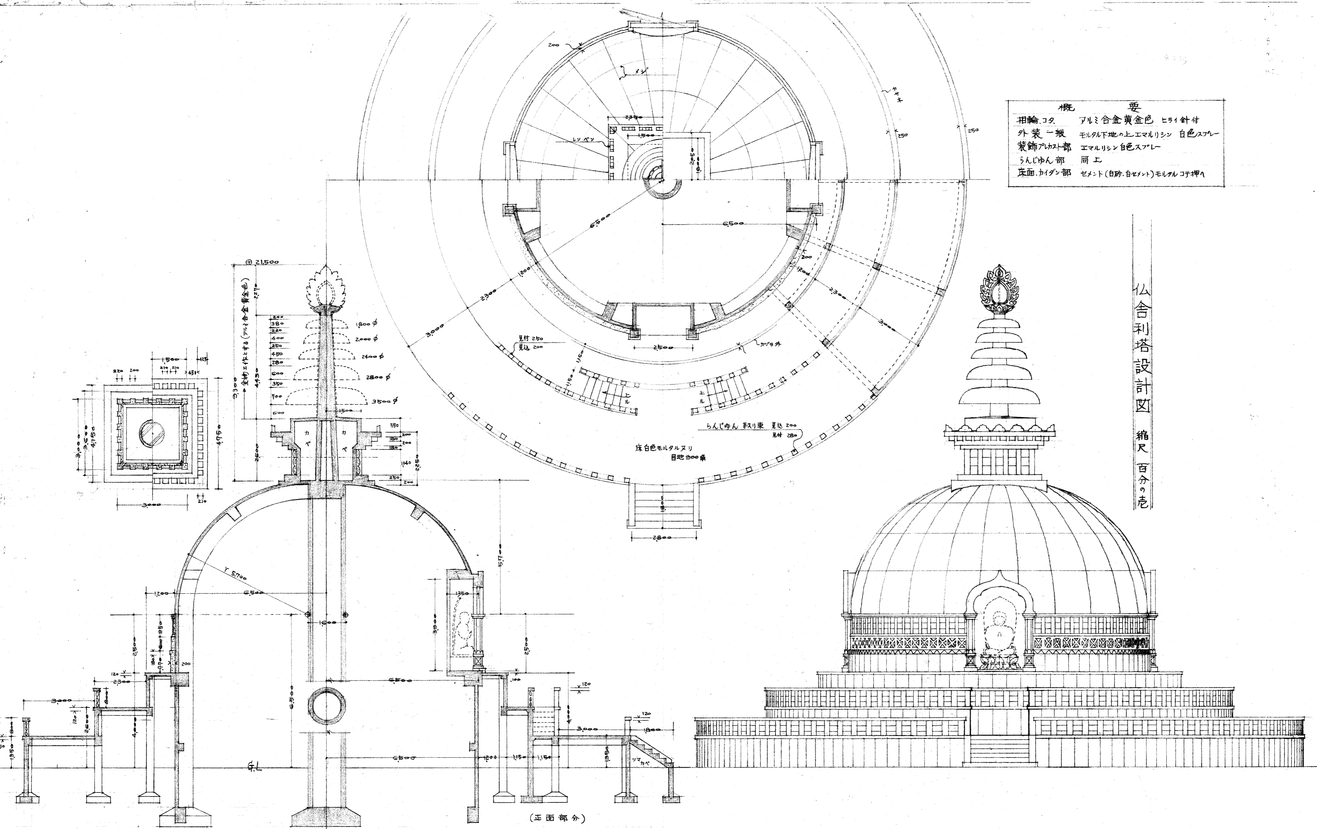
断面図 (構造寸法に関しては別図構造図参照のこと)
