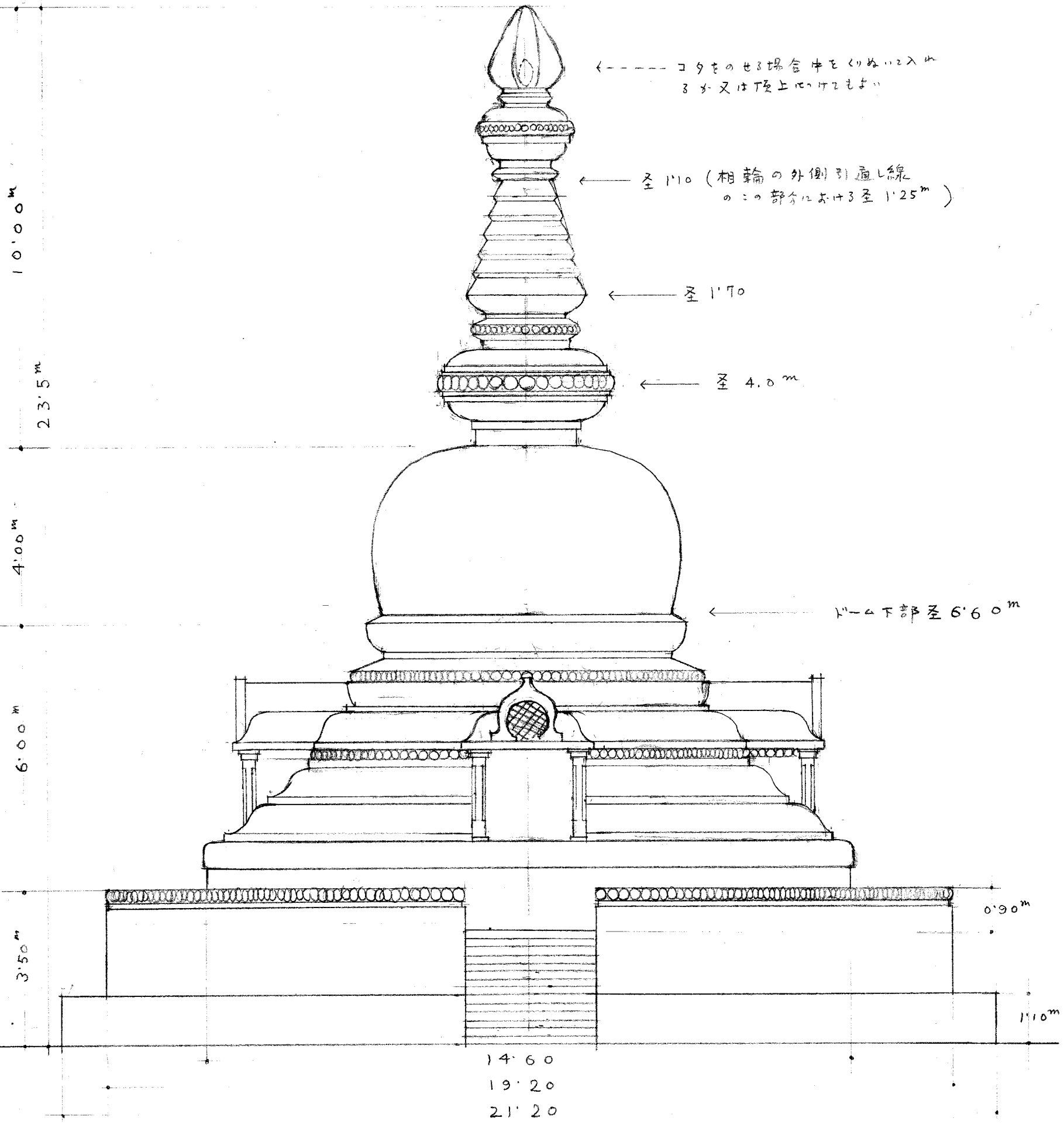
日杵仏舎利塔正立面図 5.1:100. 82.43.5.3 封
