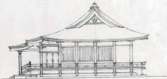
立面図
