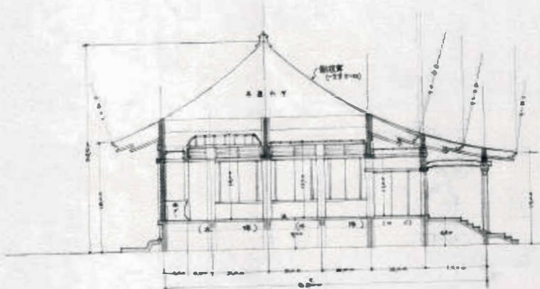
断面図 (1/100)
