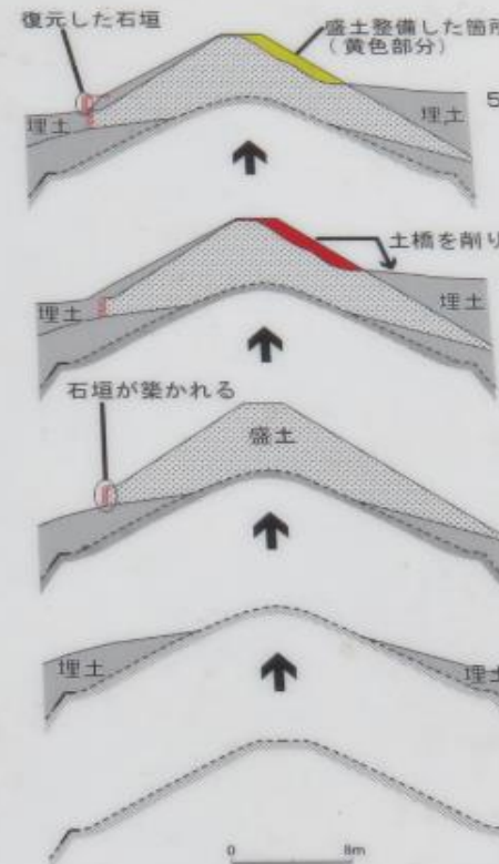
大堀切土橋変遷模式図
