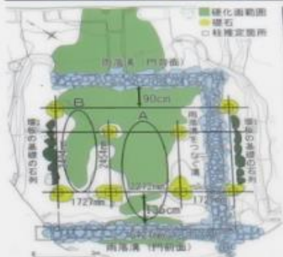
発掘調査時の郭馬出西虎口門（図面）
